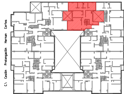
PLANTA TRASTEROS VINCULADOS
