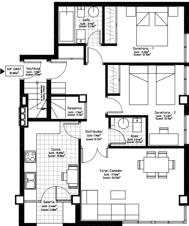
Planta Baja Modulo Tipo - Q1 -
