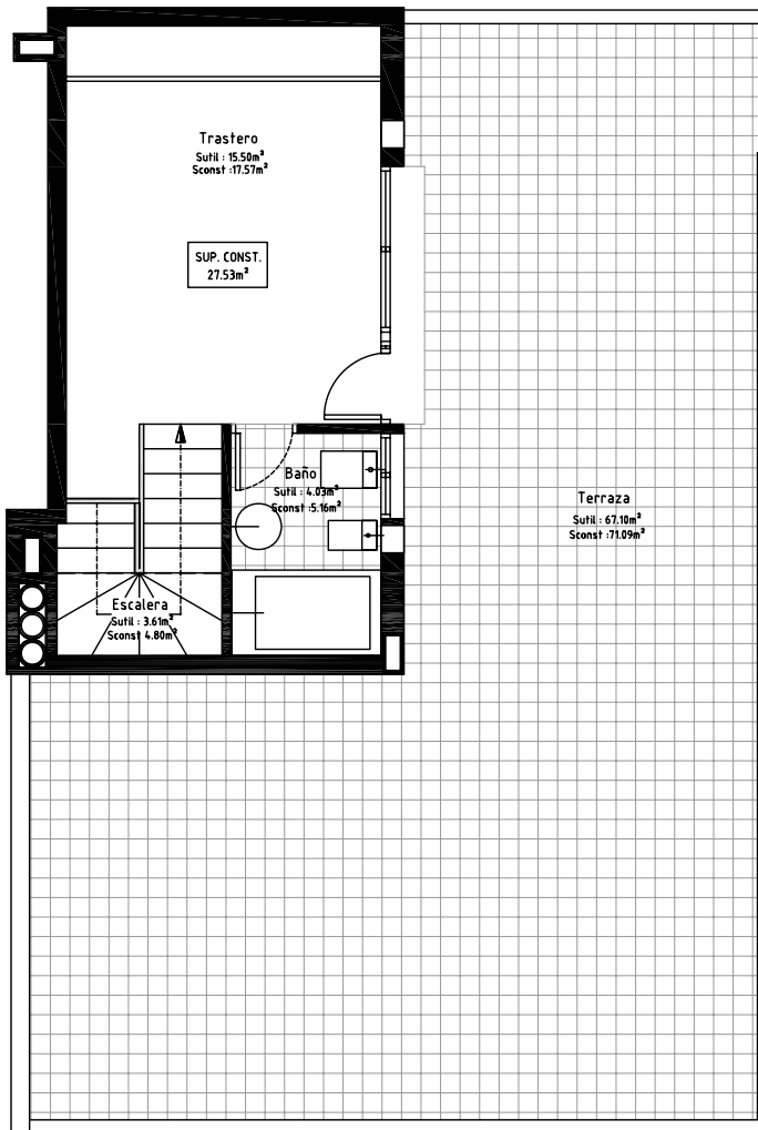
Planta Primera ( Opción de distribución ) Modulo Tipo - Q1 -
