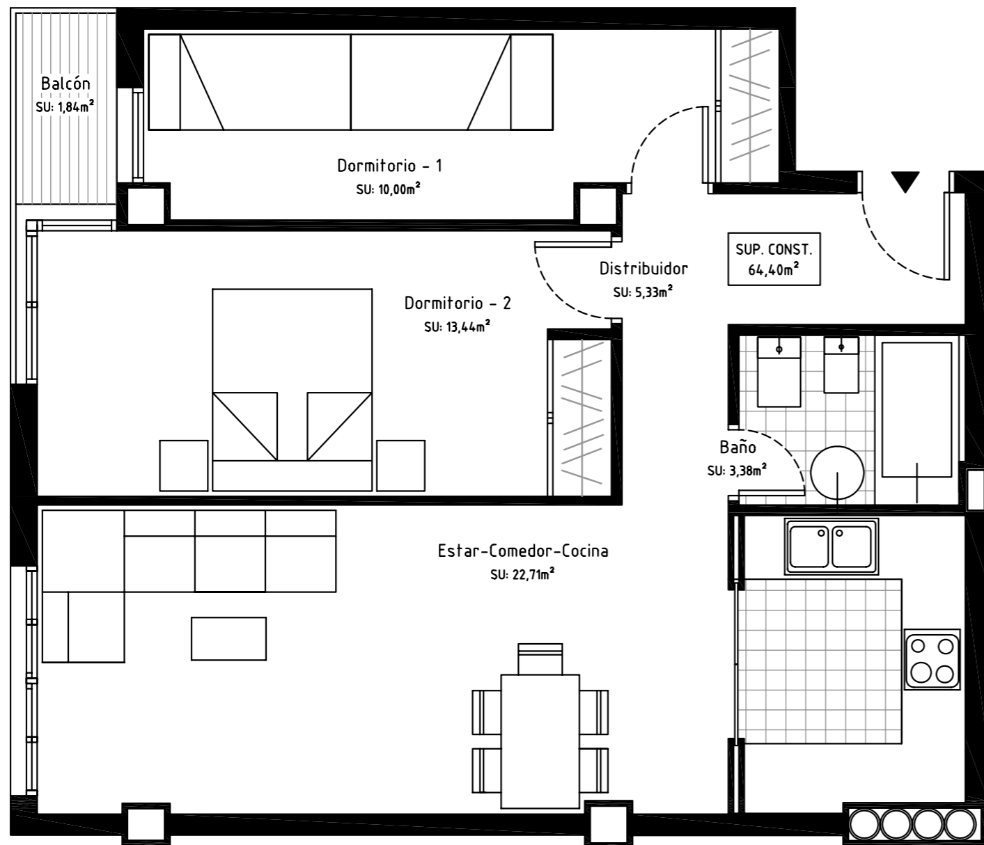
Modulo Tipo - J - ( Viviendas 25, 41 y 57 )
